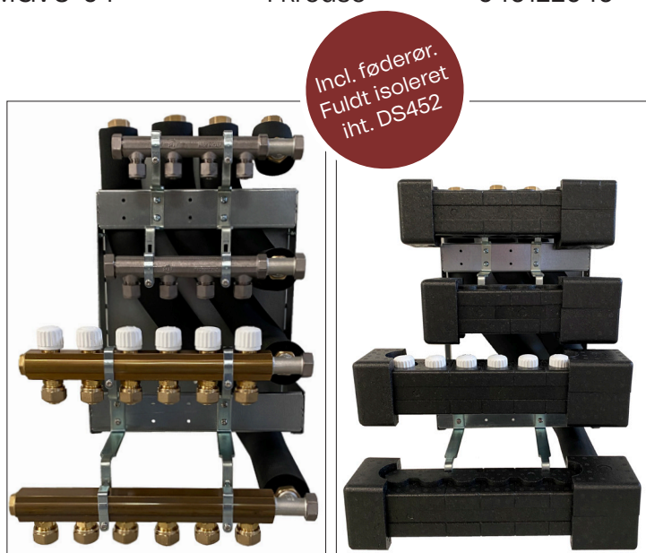
BUNDMODUL med 6 gulvvarme-, 4 koldtvands- og 4 varmtvandskredse.
