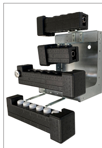
Skaktløsning med brugsvand, 5 koldtvand og 3 varmtvand. Med isolering.
