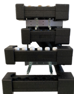
Skræddersyet BUNDMODUL med: 15 gulvvarme-, 11 koldtvands- og 8 varmtvandskredse
