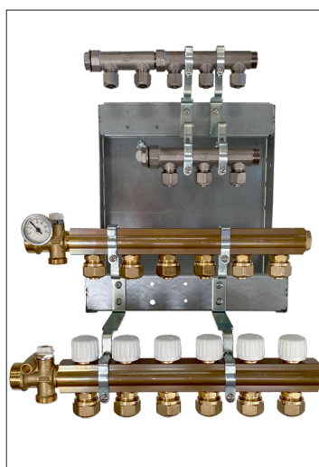
Standard skaktløsninger med 5 eller 6 gulvvarme-, 5 koldtvands- og 3 varmtvandskredse.
