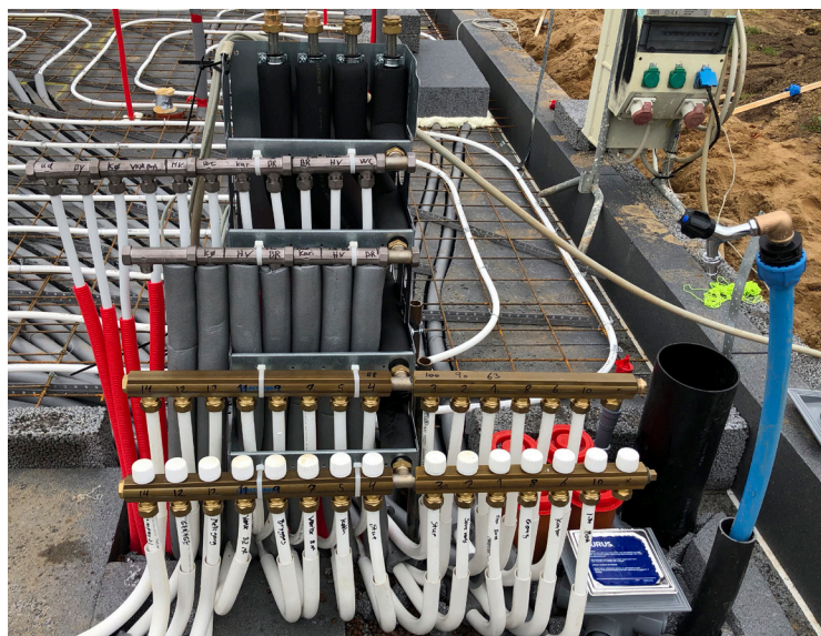
Skræddersyet BUNDMODUL med: 15 gulvvarme-, 11 koldtvands- og 8 varmtvandskredse
