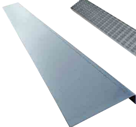
VOTEC DØRPROFIL 20x50x1000mm 1,5mm galv. stålplade. BD nr. 22 1911.505
