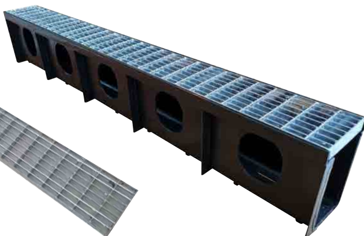
VOTEC SOKKELRIST Galvaniseret. 1000x100x20 mm. Maskestørrelse 53x10 mm. BD nr. 22 1912.100
