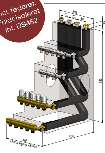
ALBE-BASICPTM: passer til flere Termix og METRO THERM fjernvarmeunits
