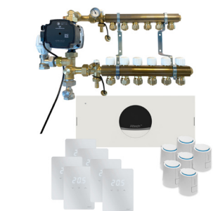
KVIKSHUNT og ALTECH PRO styring.
